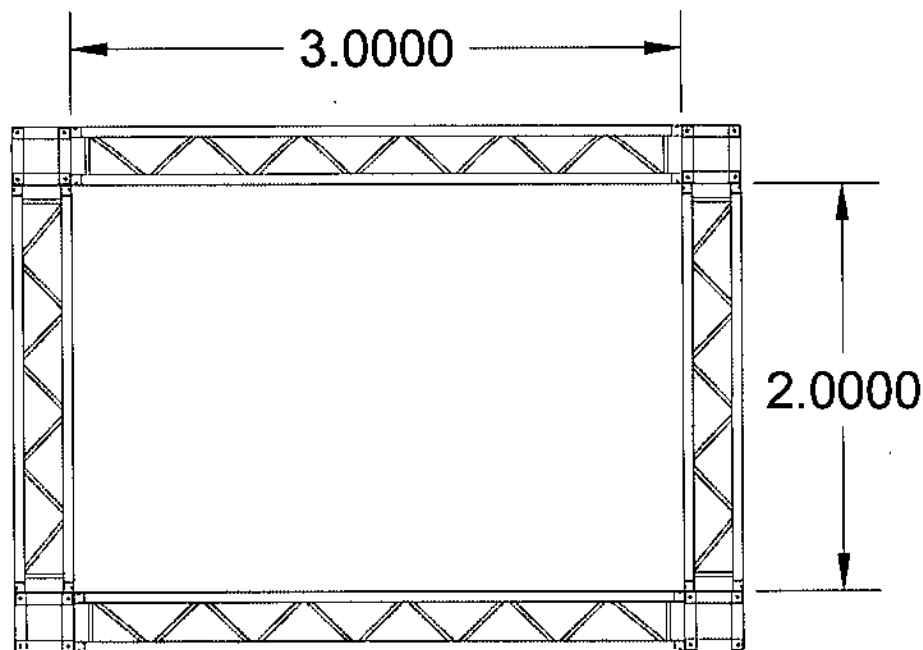
Projeto Estrutura Backdrop
