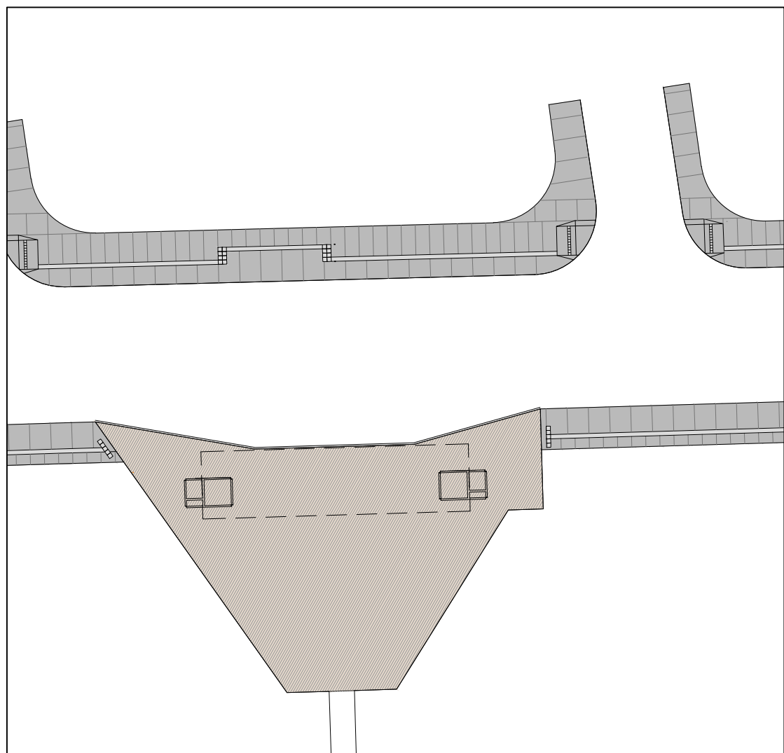
PLANTA - Q2 e Q3 - MEDIADOR B - BAL. ICARAÍ DE IGUAPE ESC. 1:500
