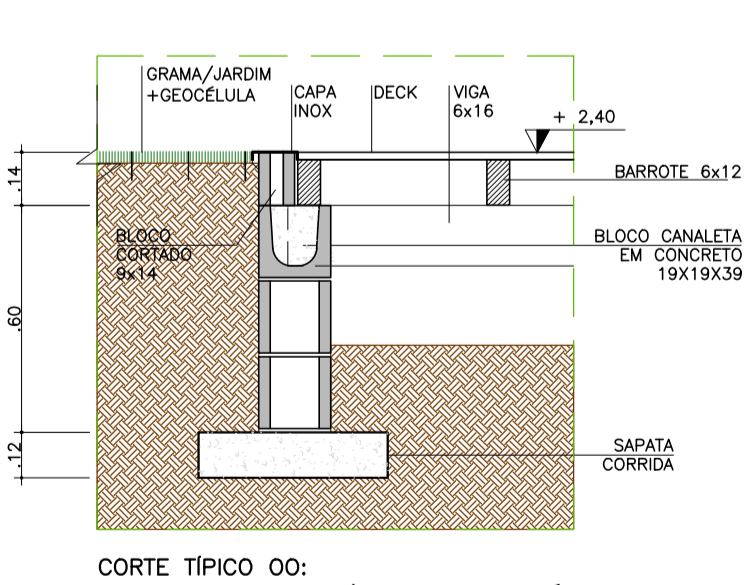
CORTE TÍPICO OO: INTERFACE DECK/GRAMA+GEOCÉLULA ESC 1/20
