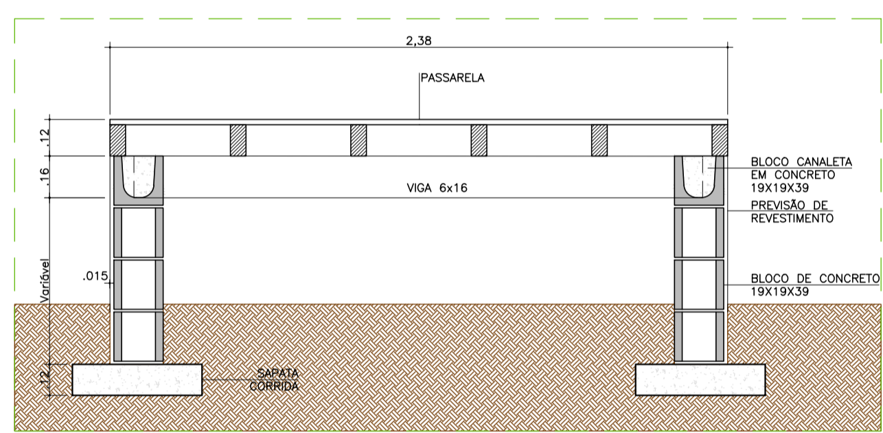
CORTE TÍPICO GG: PASSARELA ESC 1/20
