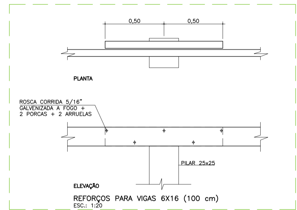
PLANTA ELEVÇÃO REFORÇOS PARA VIGAS 6X16 (100 cm) ESC: 1:20
