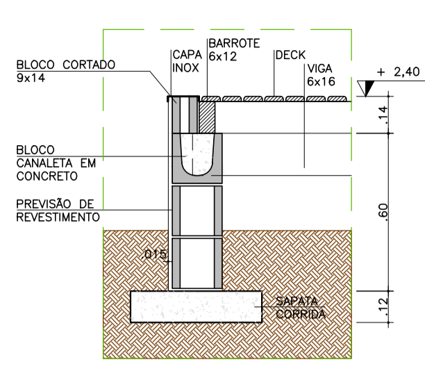
CORTE TÍPICO BB: ARREMATE DO DECK C/ PERFIL INOX ESC 1/20
