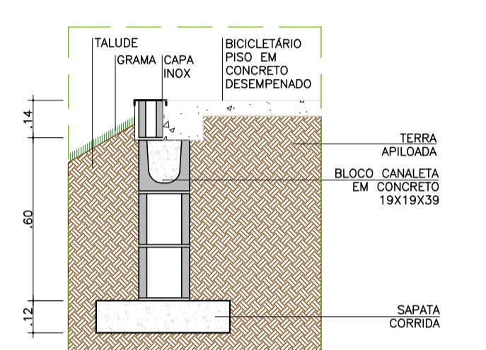
CORTE TÍPICO KK: INTERFACE TALUDE/MURO ESC 1/20
