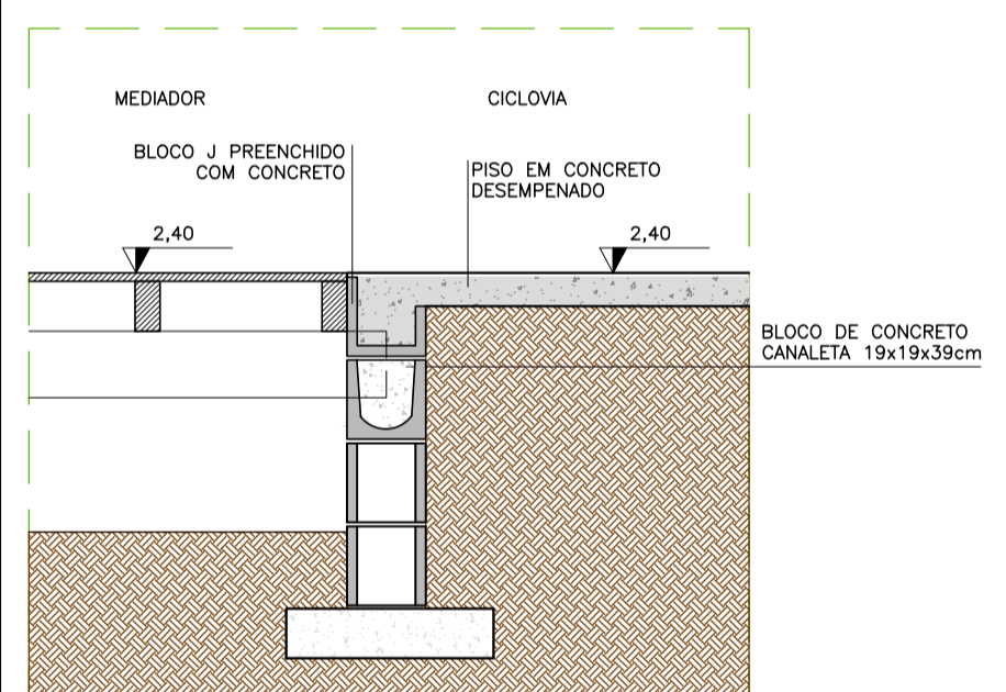
CORTE TÍPICO II: INTERFACE MURO DE ARRIMO/CICLOVIA ESC 1/20
