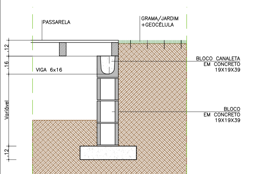
CORTE TÍPICO PP: INTERFACE PASSARELA/GRAMA+GEOCÉLULA ESC 1/20
