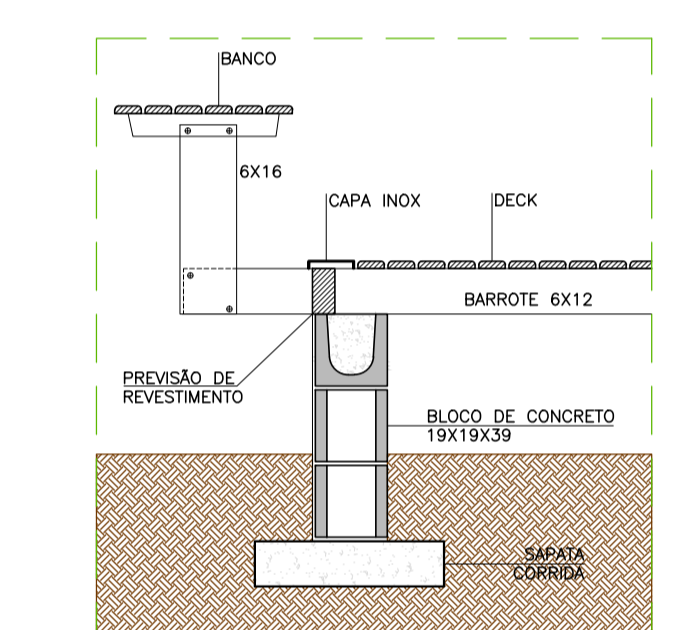
CORTE TÍPICO HH: DETALHE BANCO (MEDIADOR A) ESC 1/20
