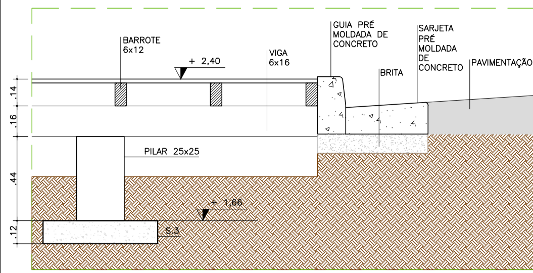
CORTE TÍPICO AA: INTERFACE DECK/AV. BEIRA MAR ESC 1/20
