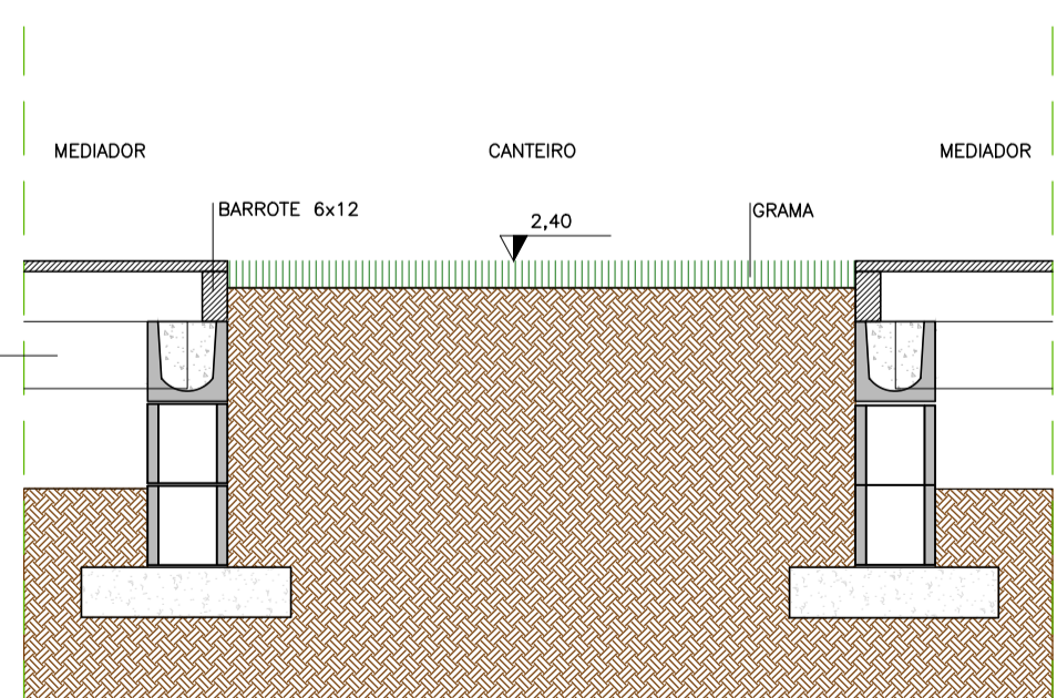
CORTE TÍPICO QQ: CANTEIRO ESC 1/20
