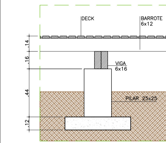
CORTE TÍPICO EE: DECK ESC 1/20
