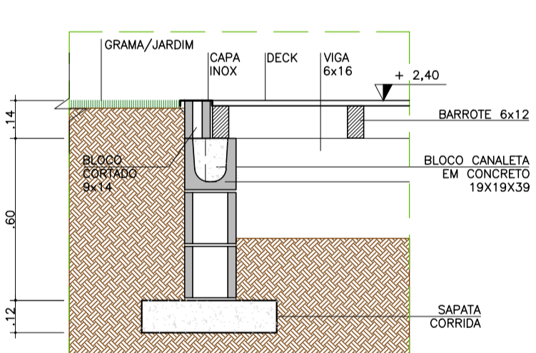
CORTE TÍPICO NN: INTERFACE DECK/GRAMA ESC 1/20
