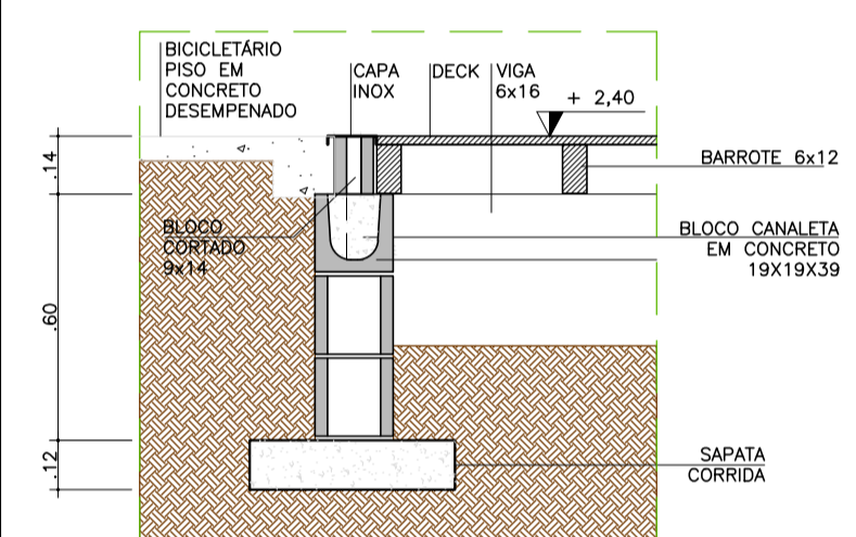
CORTE TÍPICO LL: INTERFACE BICICLETÁRIO/DECK ESC 1/20
