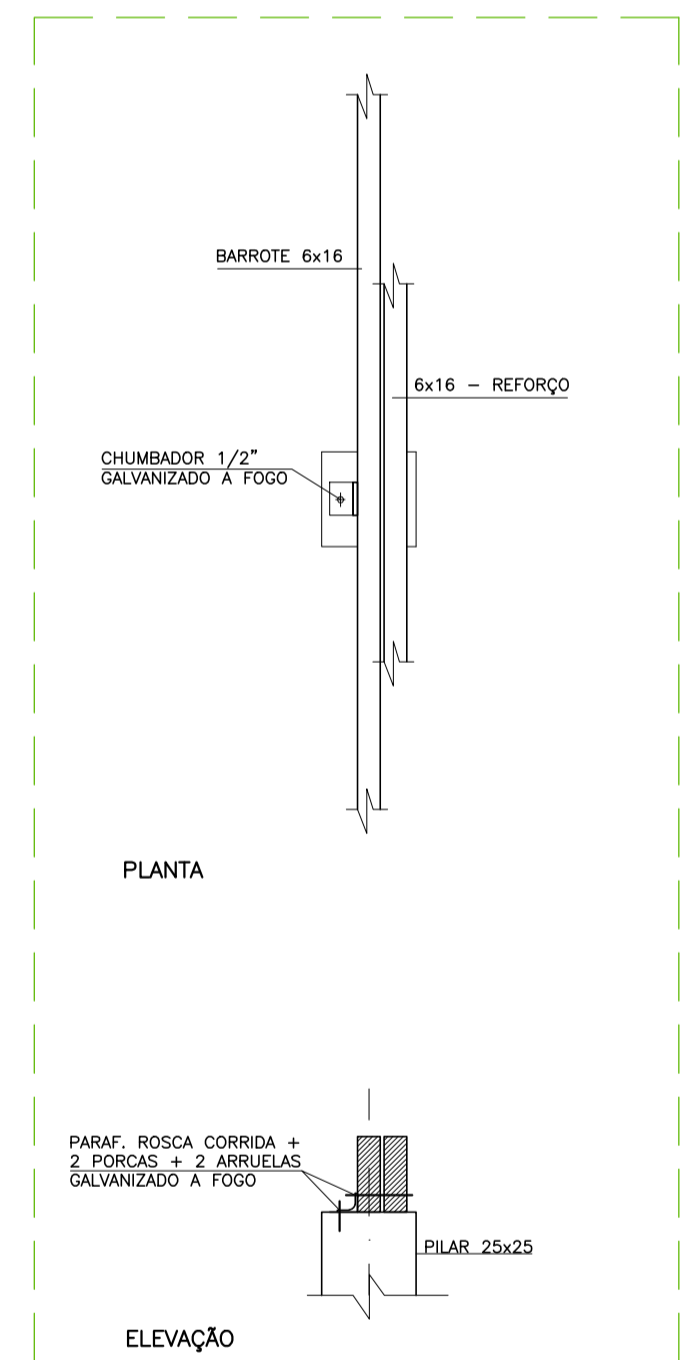
PLANTA ELEVÇÃO FIXAÇÃO VIGA X PILAR ESC: 1:20
