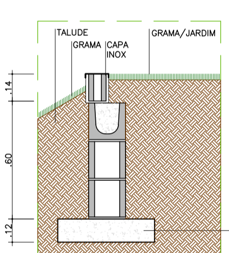
CORTE TÍPICO MM: INTERFACE TALUDE/MURO ESC 1/20
