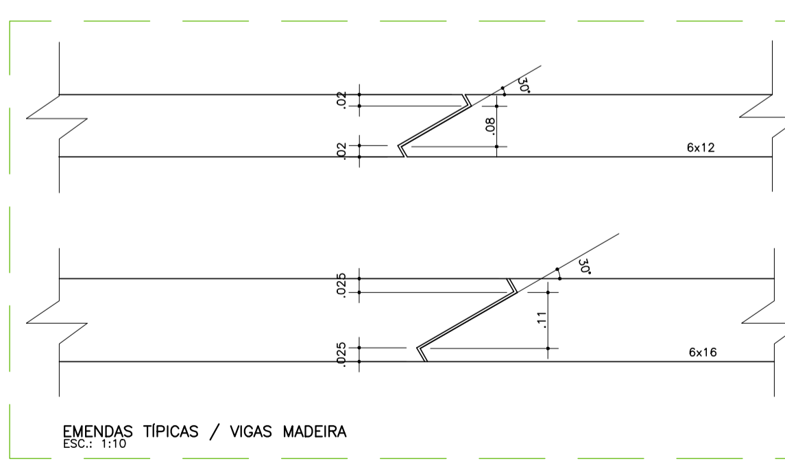
EMENDAS TÍPICAS / VIGAS MADEIRA ESC: 1:10
