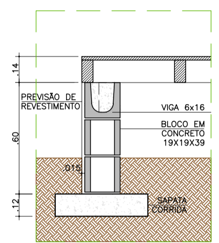
CORTE TÍPICO FF: ARREMATE DO DECK ESC 1/20
