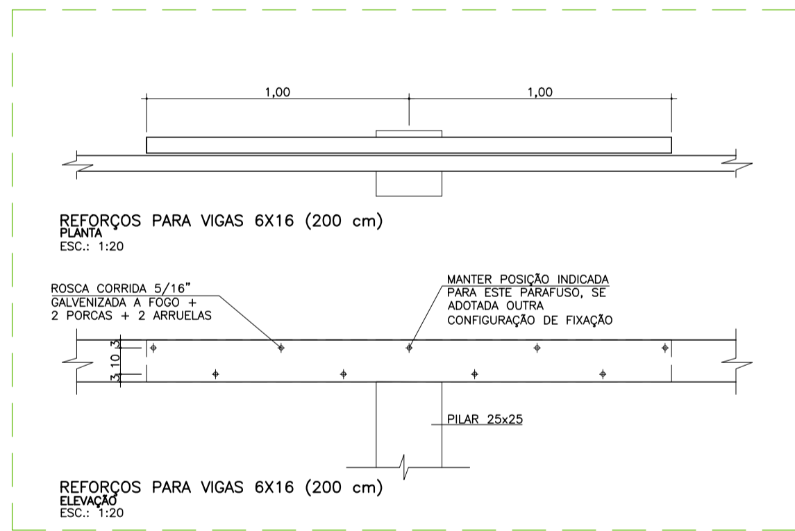
PLANTA ELEVÇÃO REFORÇOS PARA VIGAS 6X16 (200 cm) ESC: 1:20
