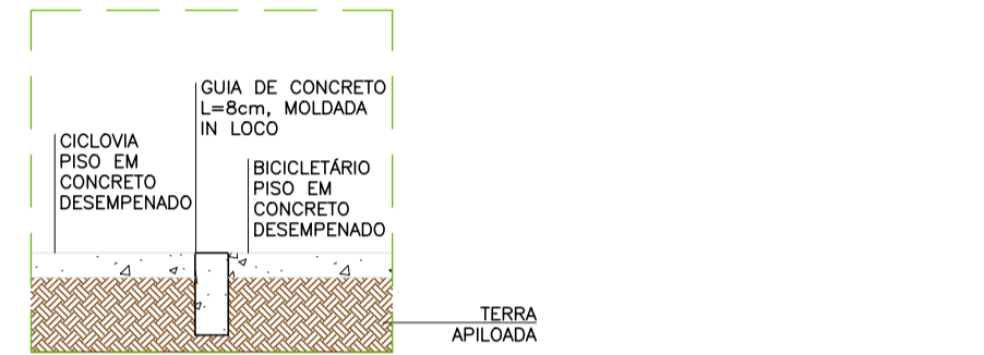
CORTE TÍPICO JJ: INTERFACE CICLOVIA/GUIA/BICICLETÁRIO ESC 1/20
