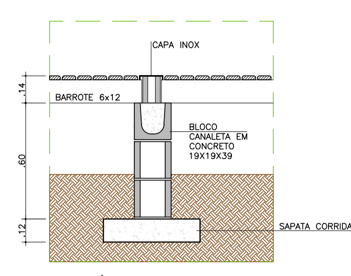
CORTE TÍPICO DD: INTERFACE MADEIRA/INOX/MADEIRA ESC 1/20
