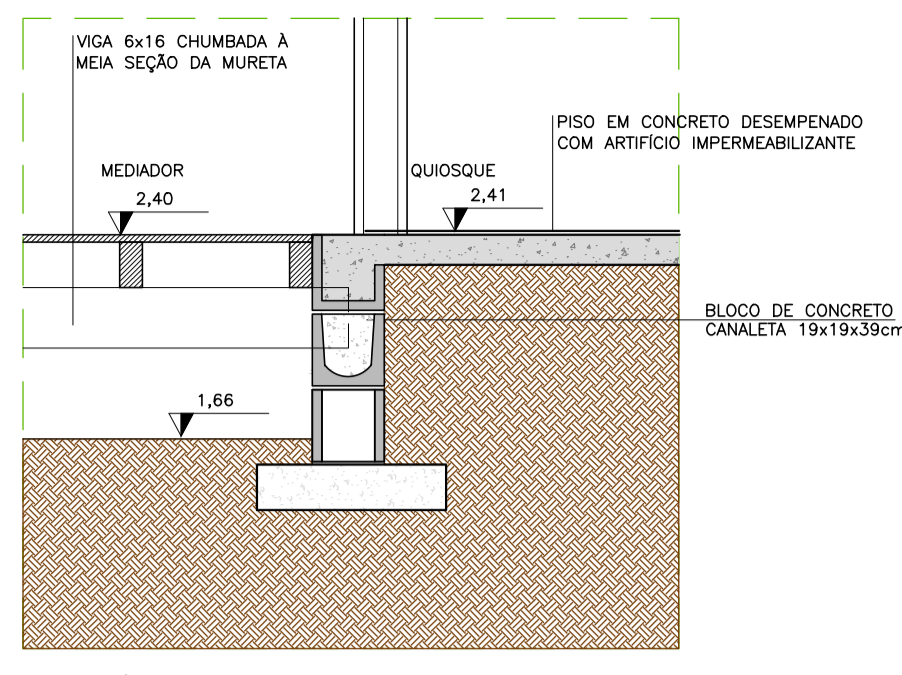
CORTE TÍPICO CC: INTERFACE MURETA/QUIOSQUE ESC 1/20
