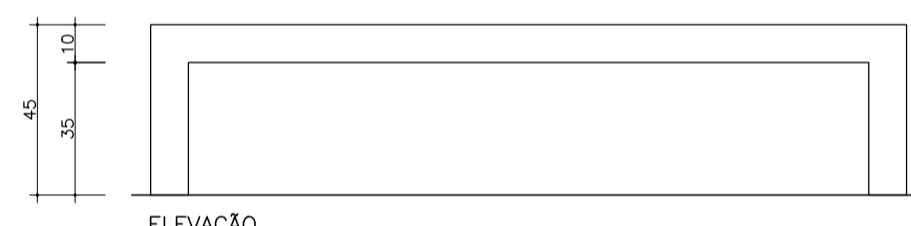
ELEVAÇÃO
