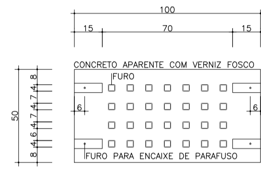
PLANTA – VISTA INFERIOR
