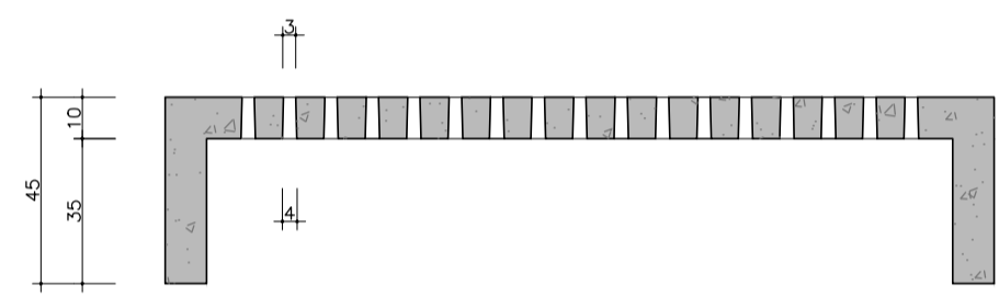
CORTE LONGITUDINAL
