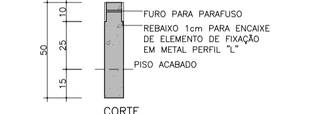
CORTE
