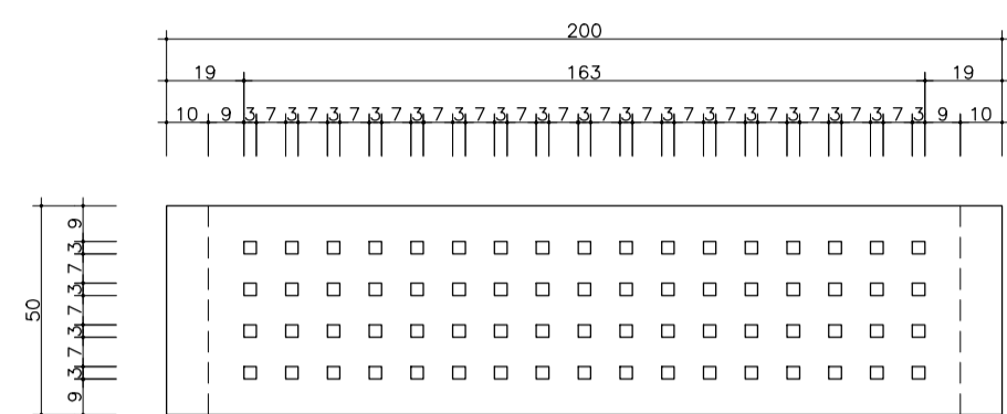
PLANTA – VISTA SUPERIOR
