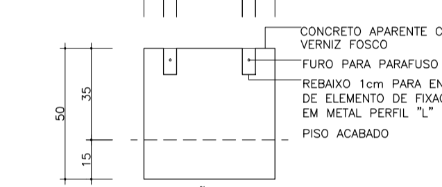
ELEVAÇÃO 01
