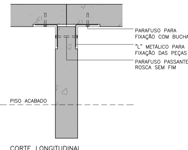
CORTE LONGITUDINAL
