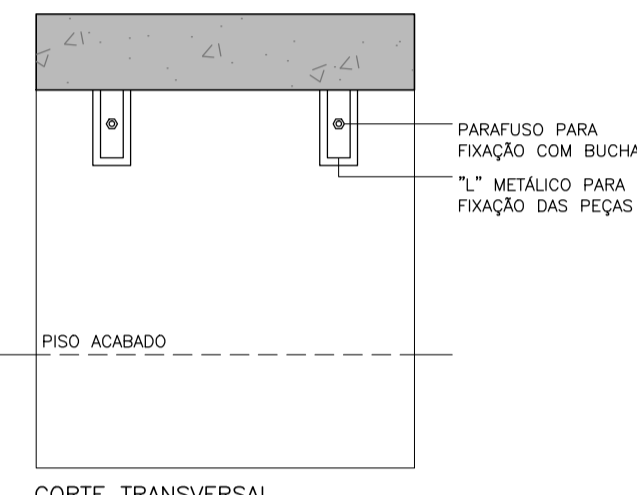
CORTE TRANSVERSAL
