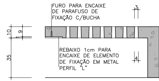
CORTE LONGITUDINAL
