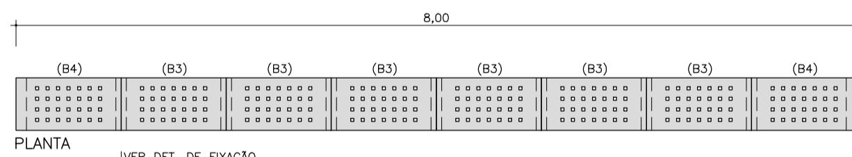
PLANTA
