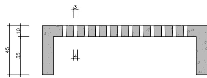
CORTE LONGITUDINAL
