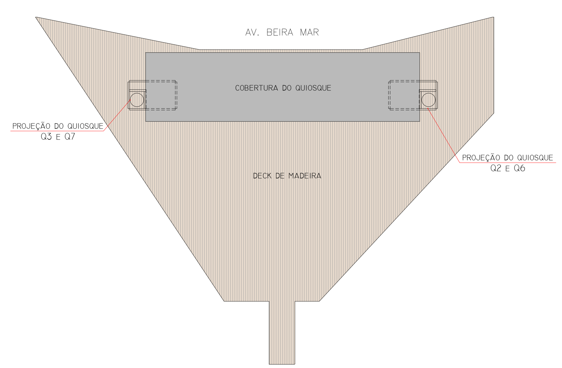
IMPLANTAÇÃO NO MEDIADOR B ESCALA 1:500
